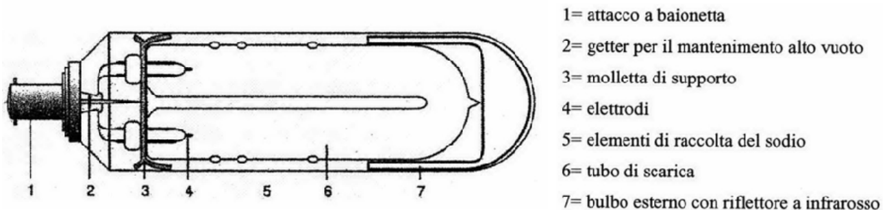
Figura 6.5 - lampada a vapori di sodio a bassa pressione
