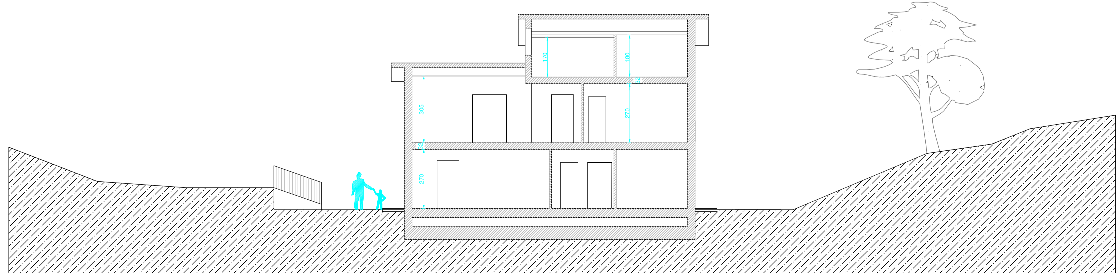
SEZIONE LONGITUDINALE C - C'
