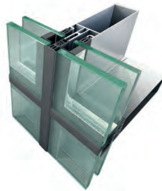
Sezione facciata continua Ponzi | Detail curtain wall
