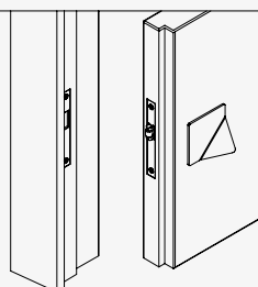
Serratura con scrocco a rullo con maniglia tira porta TRI-HANDLE
