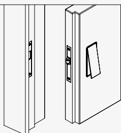
Serratura con scrocco a rullo con leva tira porta a incasso LARGE
