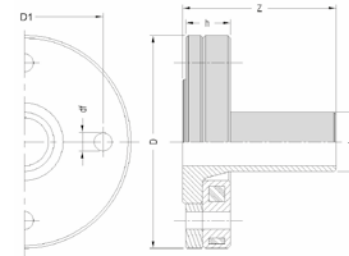
tipo B - cartella, flangia acciaio rivestita PP e anello PP
