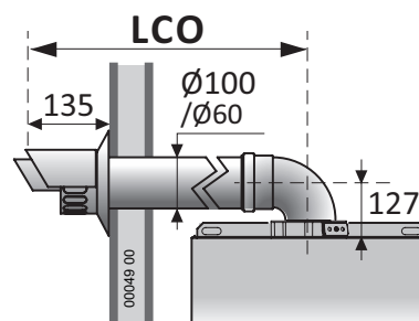
Esempio di sistema coassiale orizzontale (C 13 )
